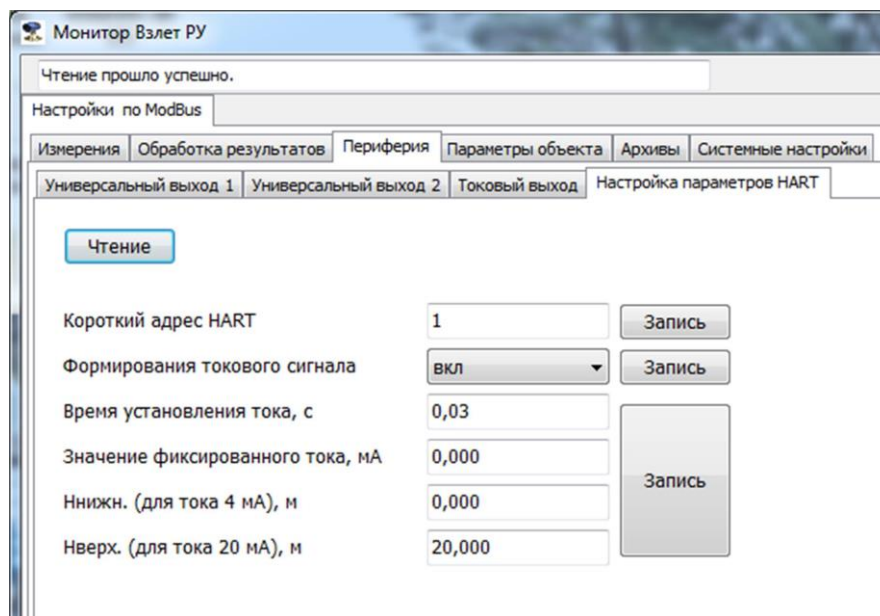
Рис.19 - Вкладка «Периферия / Настройка параметров HART».
