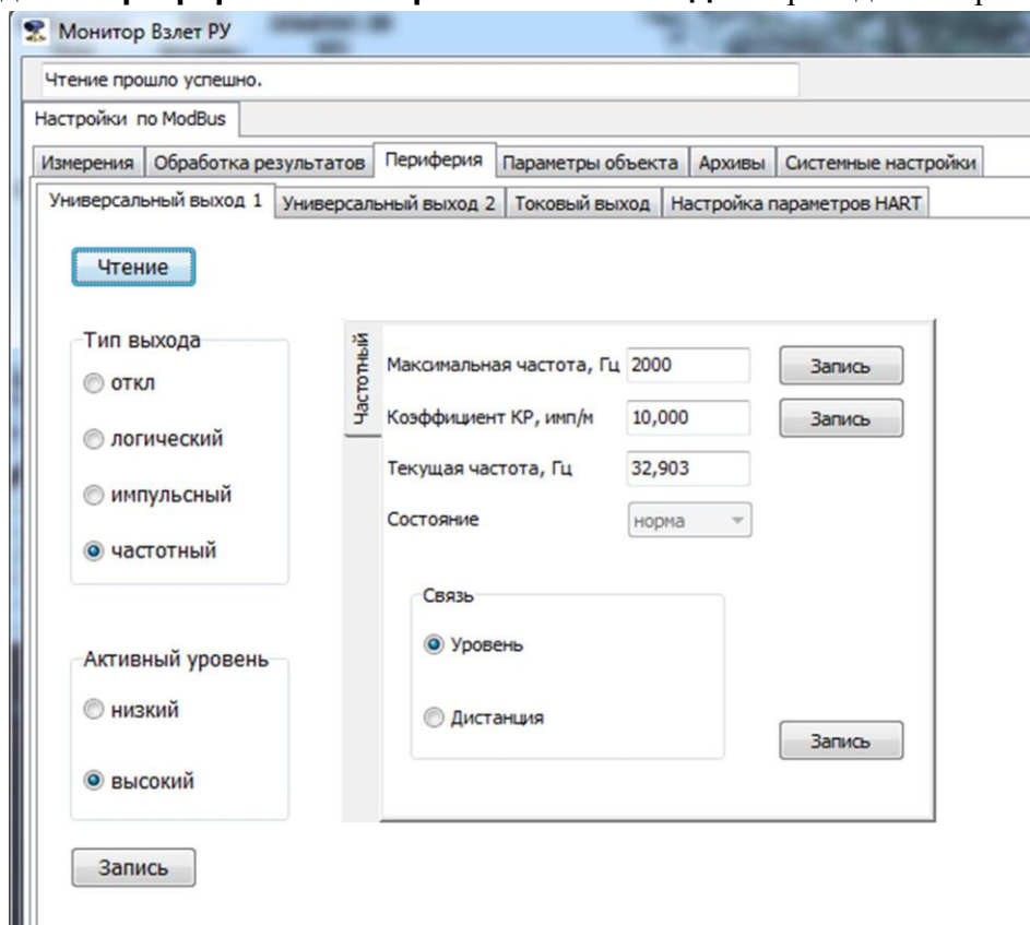
Рис.17 - Вкладка «Периферия / Универсальный выход 1».
