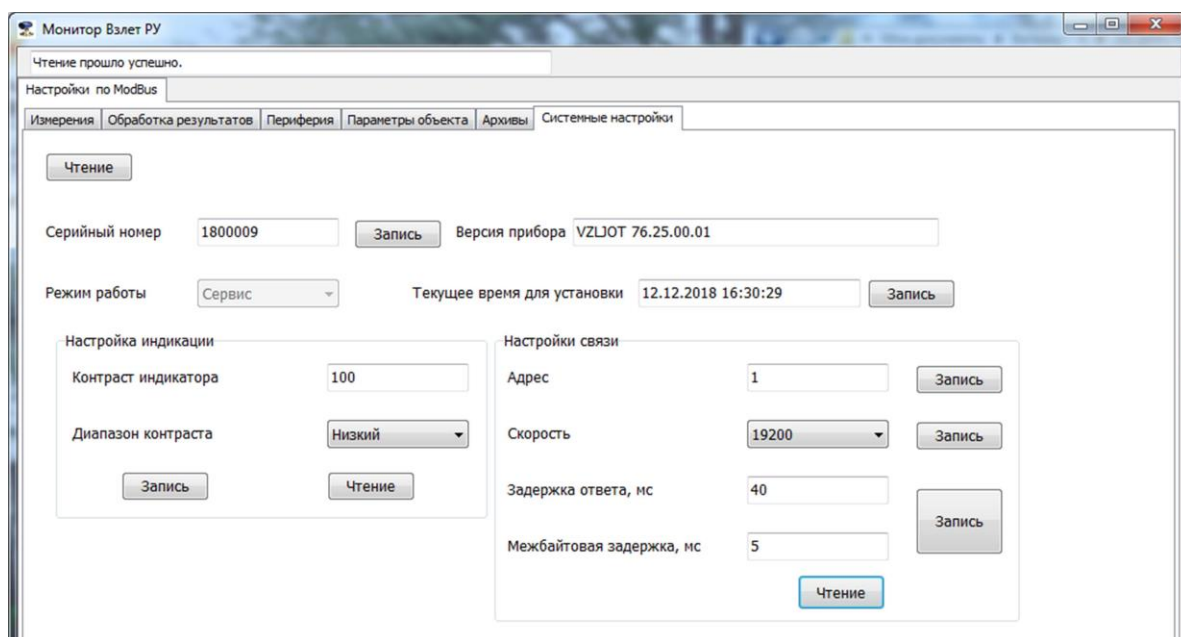
Рис.16 - Вкладка « Системные настройки ».
