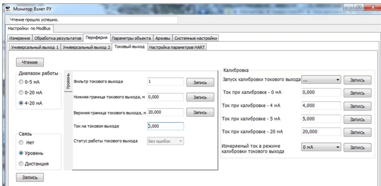
Рис.18 - Вкладка «Периферия / Токовый выход».
